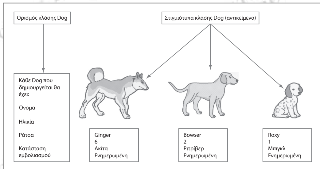
Εικόνα 1-2 Ορισμός κλάσης Dog και ορισμένα αντικείμενα που δημιουργούνται απ' αυτήν
